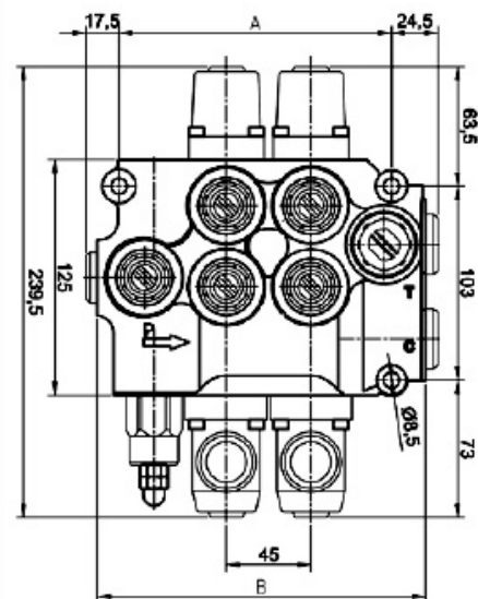
DISTRIBUIDOR 1 a 3 MANDOS 1/2" TIPO I
