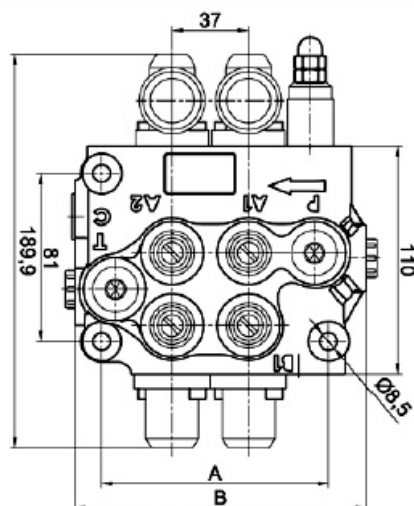
DISTRIBUIDOR 1 a 6 MANDOS 3/8" TIPO H
