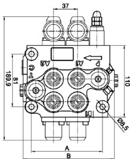
DISTRIBUIDOR 1 a 6 MANDOS 3/8" TIPO H
