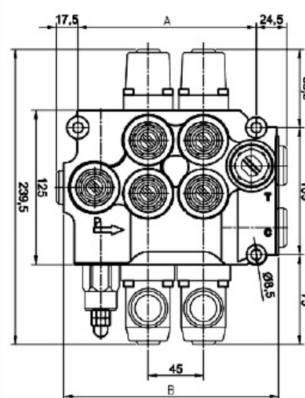
DISTRIBUIDOR 1 a 3 MANDOS 1/2" TIPO I
